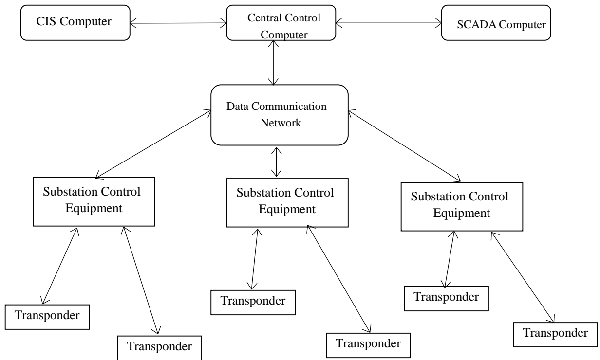
TWACS AMR 架構圖
