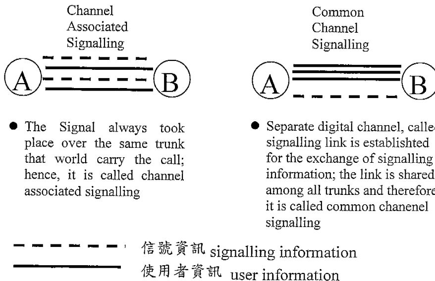
圖二、兩種信號方式的差異
