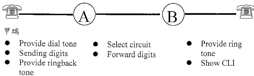
圖一、信號運作的簡例說明
