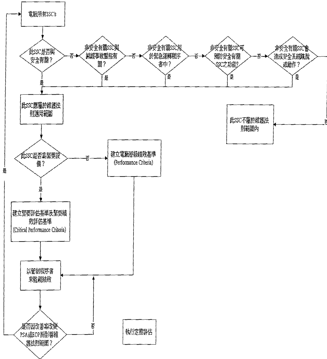
圖九 維護法則實行流程圖
