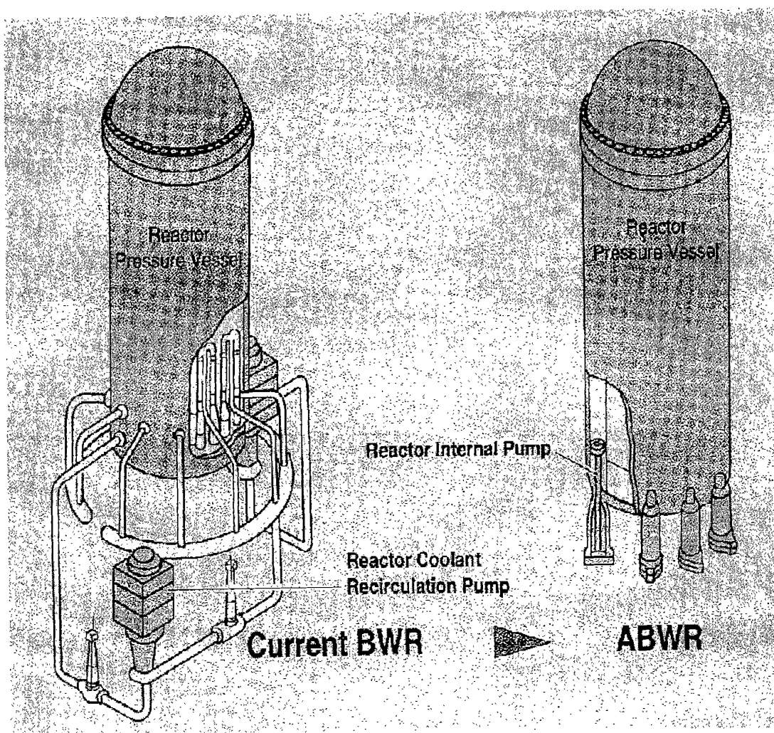
圖一 現行 BWR 與 ABWR 之比較
