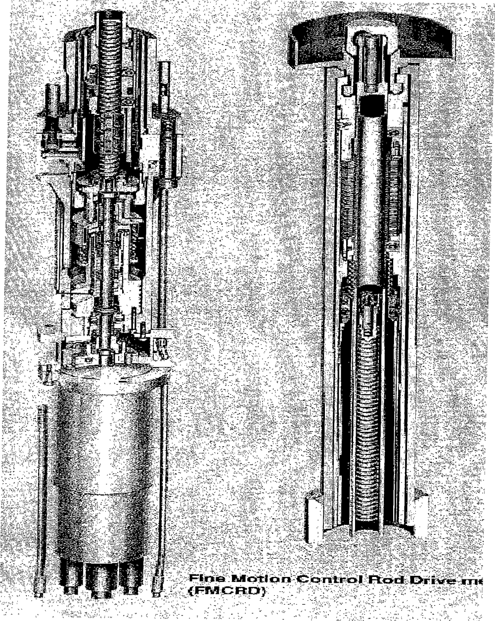
圖四 微調控制棒驅動機構剖面圖
