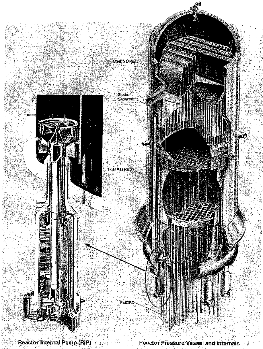
圖五 RIP位置及剖面圖
