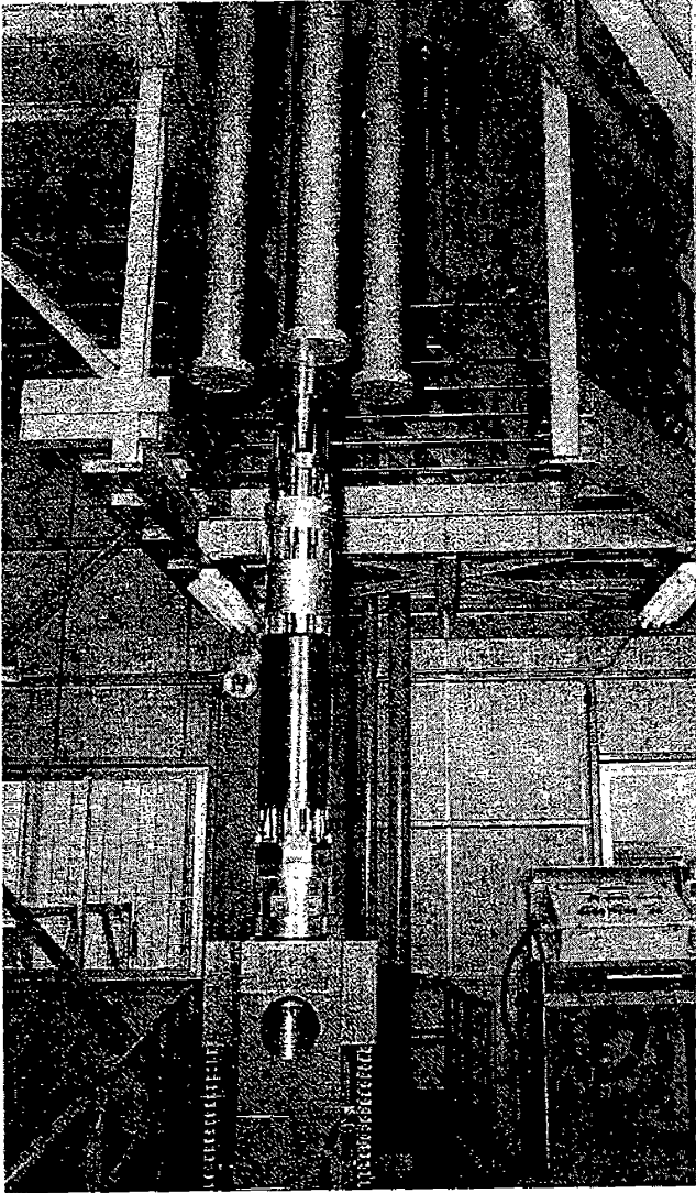
圖七 FMCRD維修訓練設備實體模型
