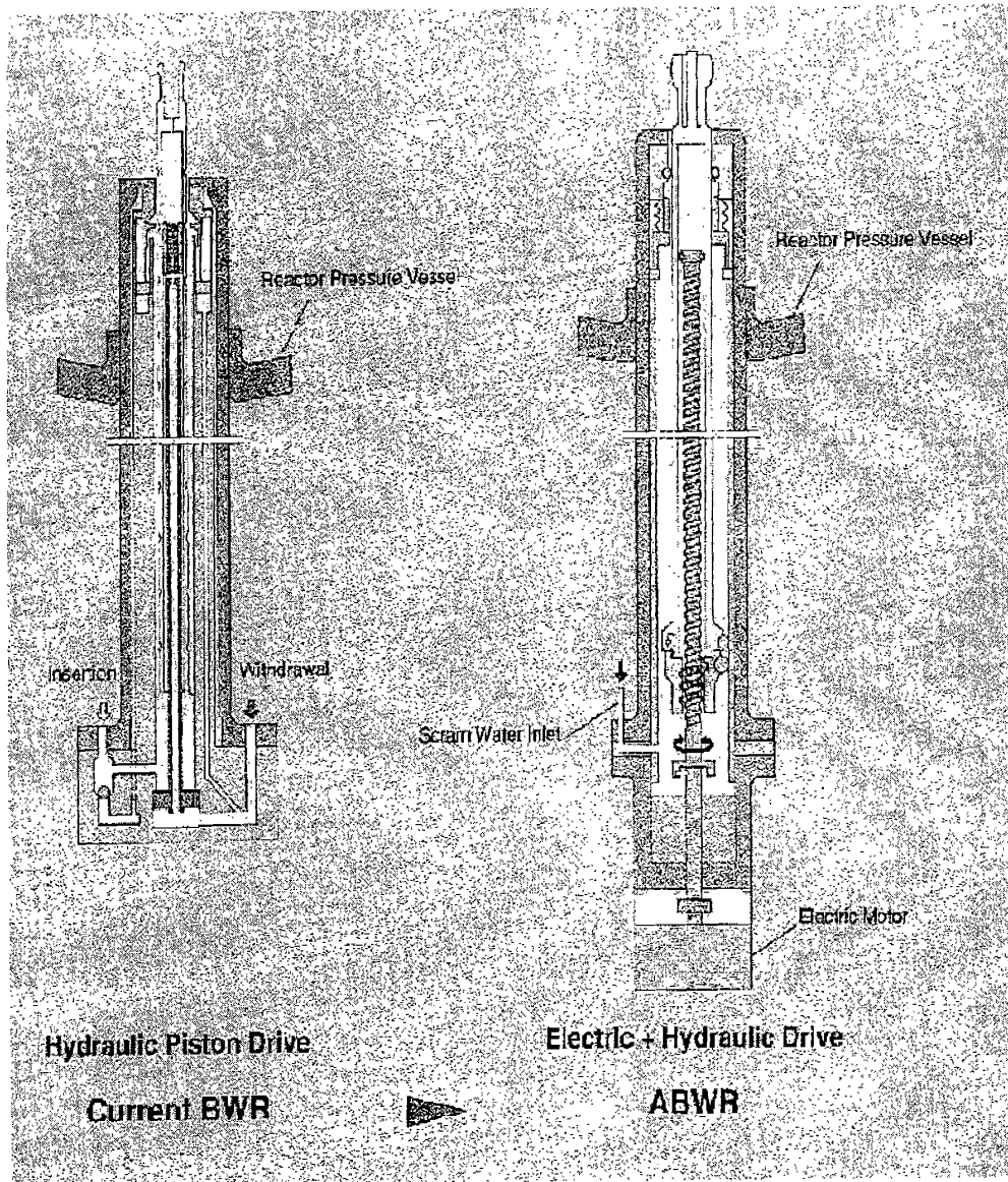
圖二 傳統CRD與FMCRD之比較
