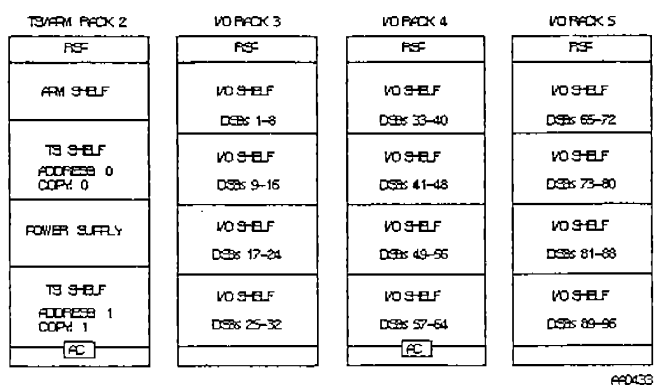
圖 3.2 典型的機架配置
