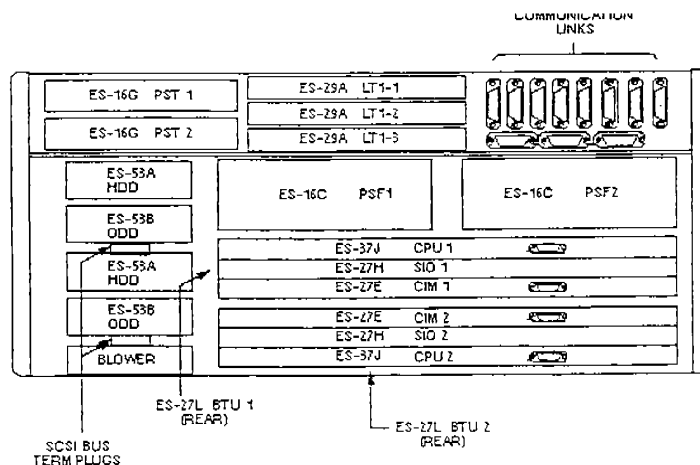
圖 3.5 AMP 時槽機框組
