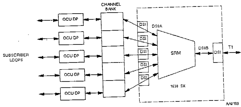
圖 3.11 Subrate Services 功能應用
